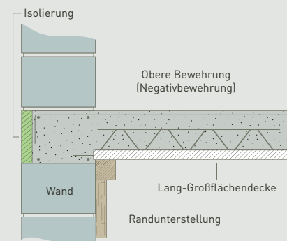
Auflagerausbildung (Mauerwerk) mit Randunterstellung
