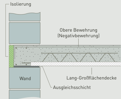
Auflagerausbildung (Mauerwerk) ohne Randunterstellung
